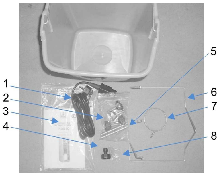
Рисунок 4 — Комплектующие, входящие в комплект поставки.
