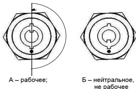
Рисунок 37 — программирование замка Mizmatic.
