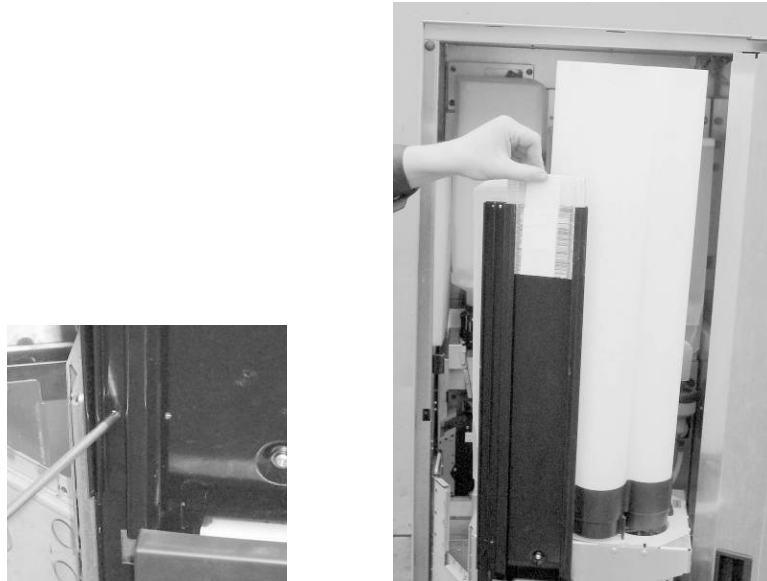
Рисунок 18 — обслуживание диспенсера размешивателей.
