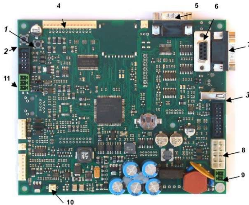
Рисунок 32 — плата управления (контроллер).
