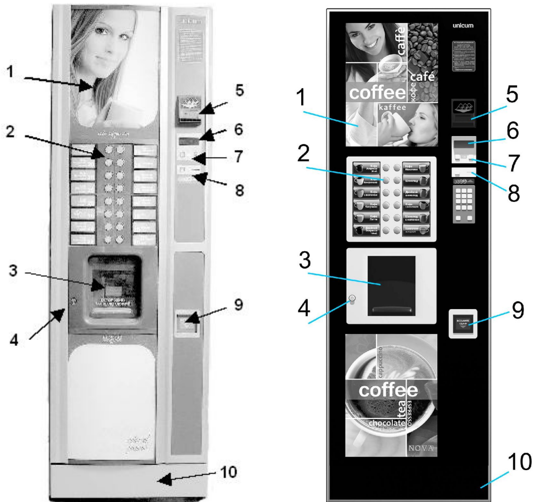
Рисунок 6 — Внешний вид автомата (слева ROSSO, справа NOVA).
